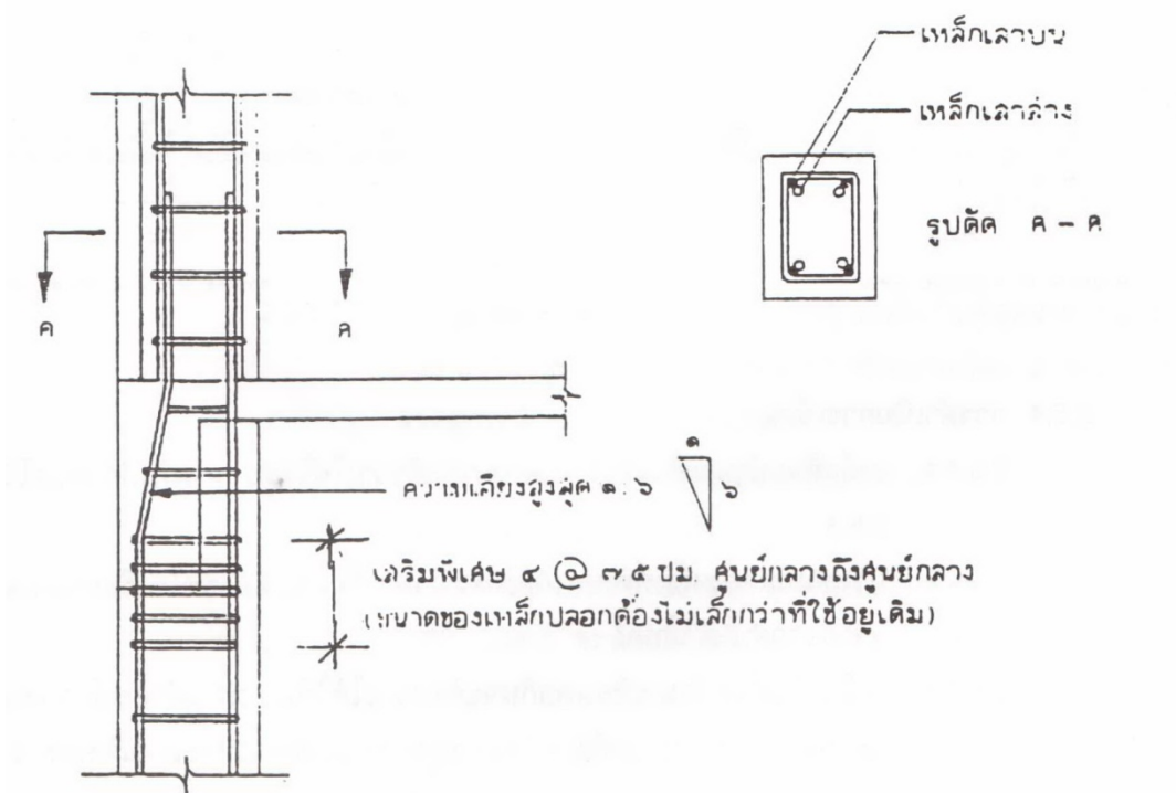
รูป กรณีเสามีหน้าตัดไม่เท่ากันศูนย์เยื้องกัน
