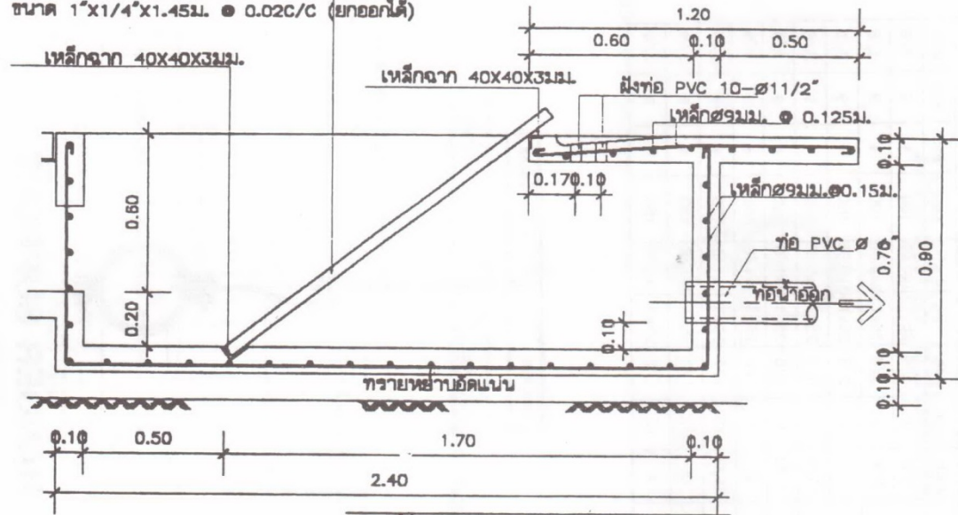
รูปตัด B-B 1 : 20
