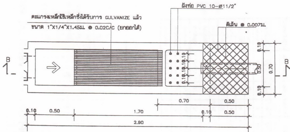
ปอดักขยะ 1 : 20
