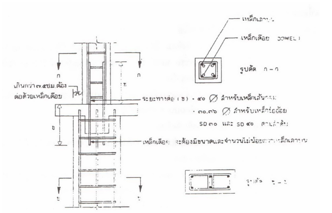
รูป กรณีเสามีหน้าตัดไม่เท่ากันศูนย์ตรงกัน
