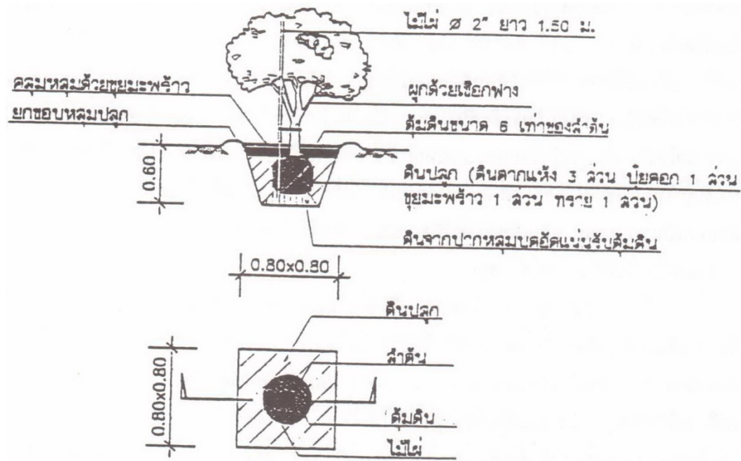
แบบรายละเอียดการปลูกต้นไม้ขนาดเล็ก
