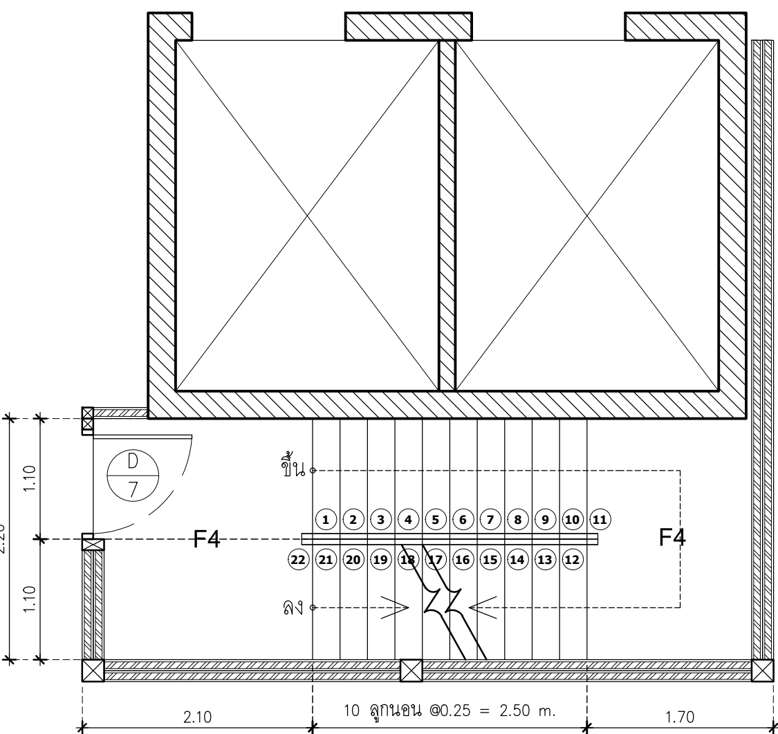
แปลนขยายบันได ST-12
