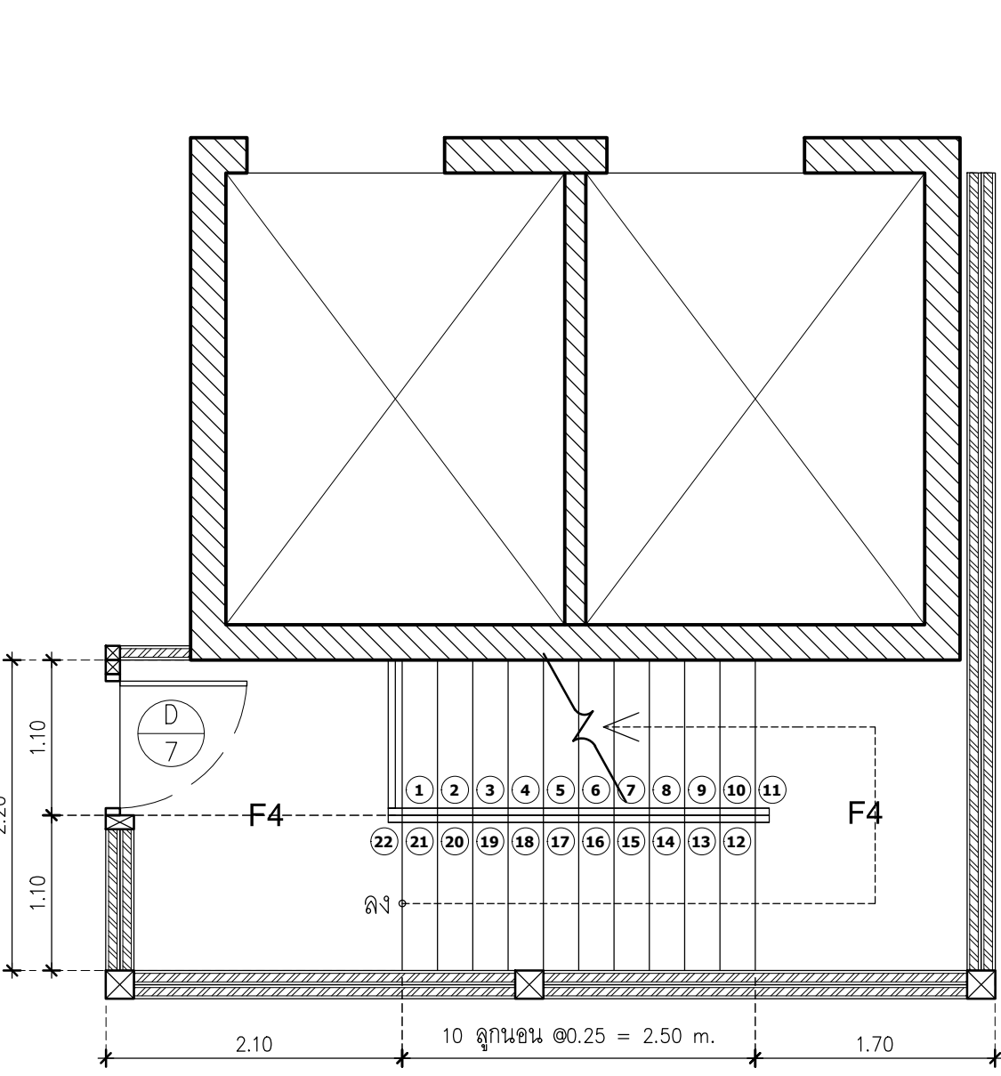
แปลนขยายบันได ST-12
