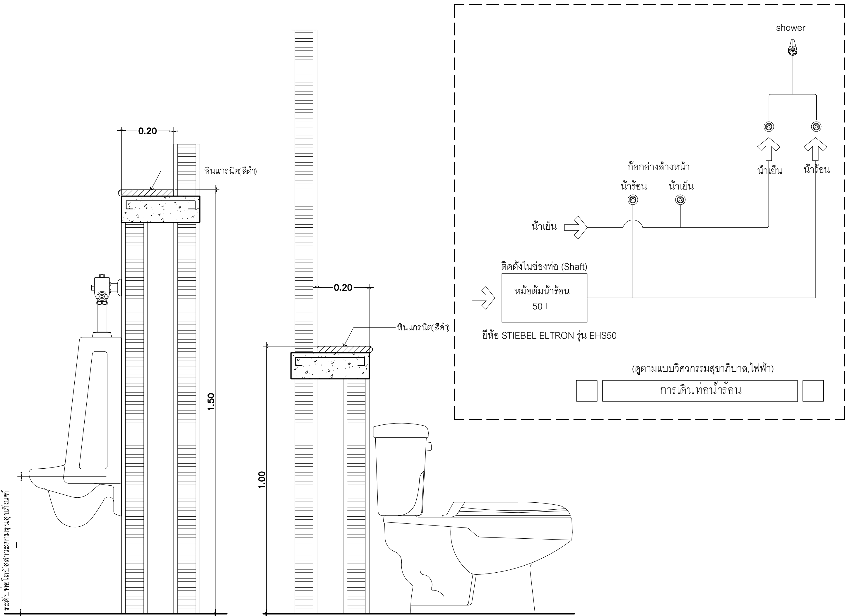
แบบขยายติดตั้งโถปัสสาวะ (ห้องน้ำสาธารณะ) มาตรฐาน
