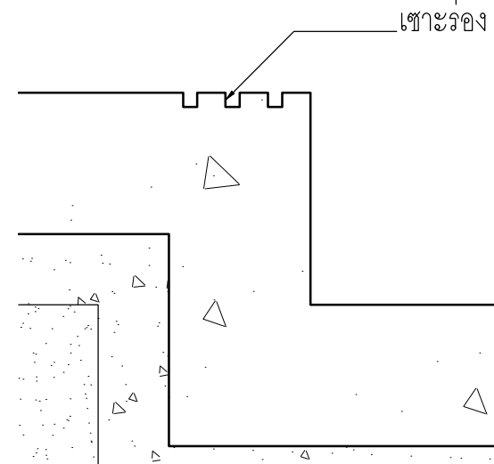
แบบขยายจุมุกบันได ST-8
