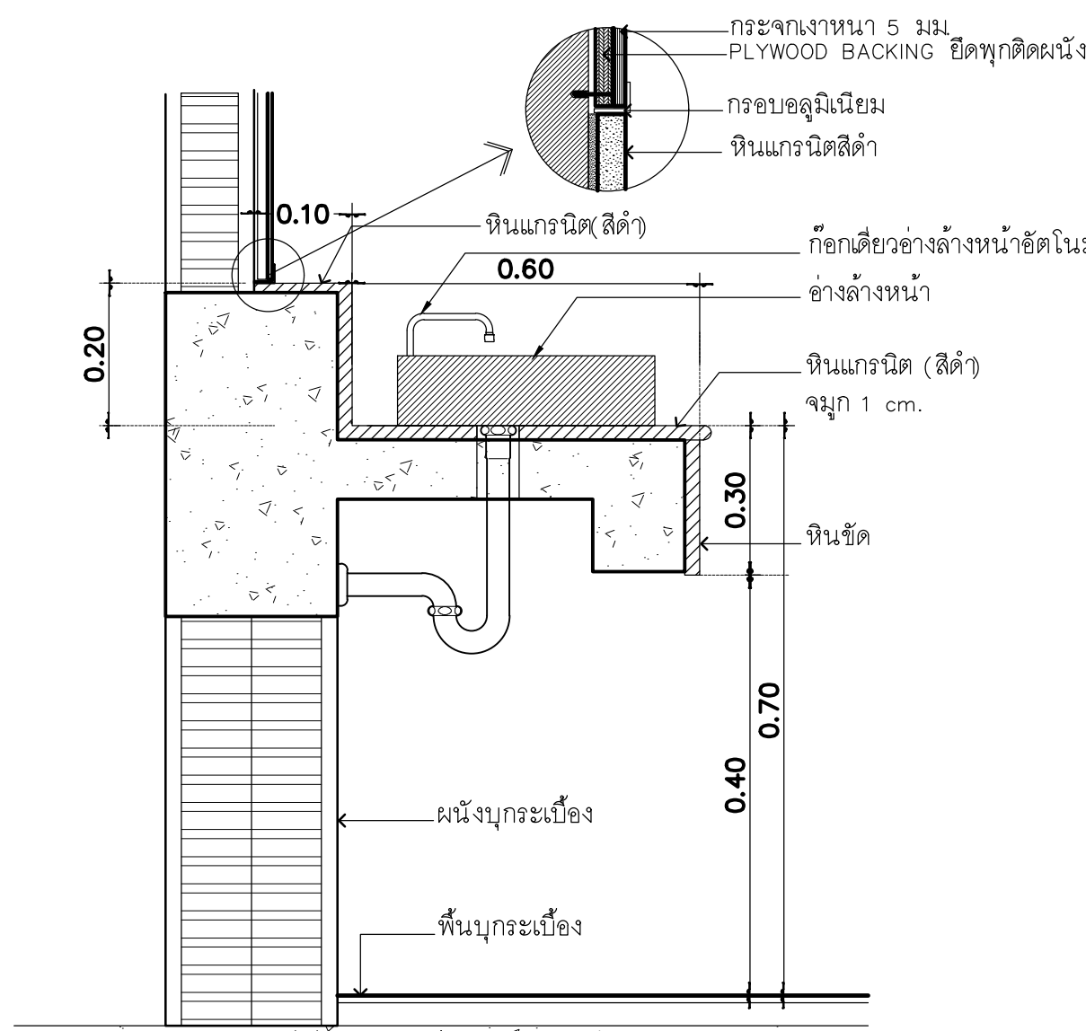
แบบขยายเคาน์เตอร์อ่างล้างหน้า (ห้องน้าสาธารณะ) มาตรฐาน 1 : 10
