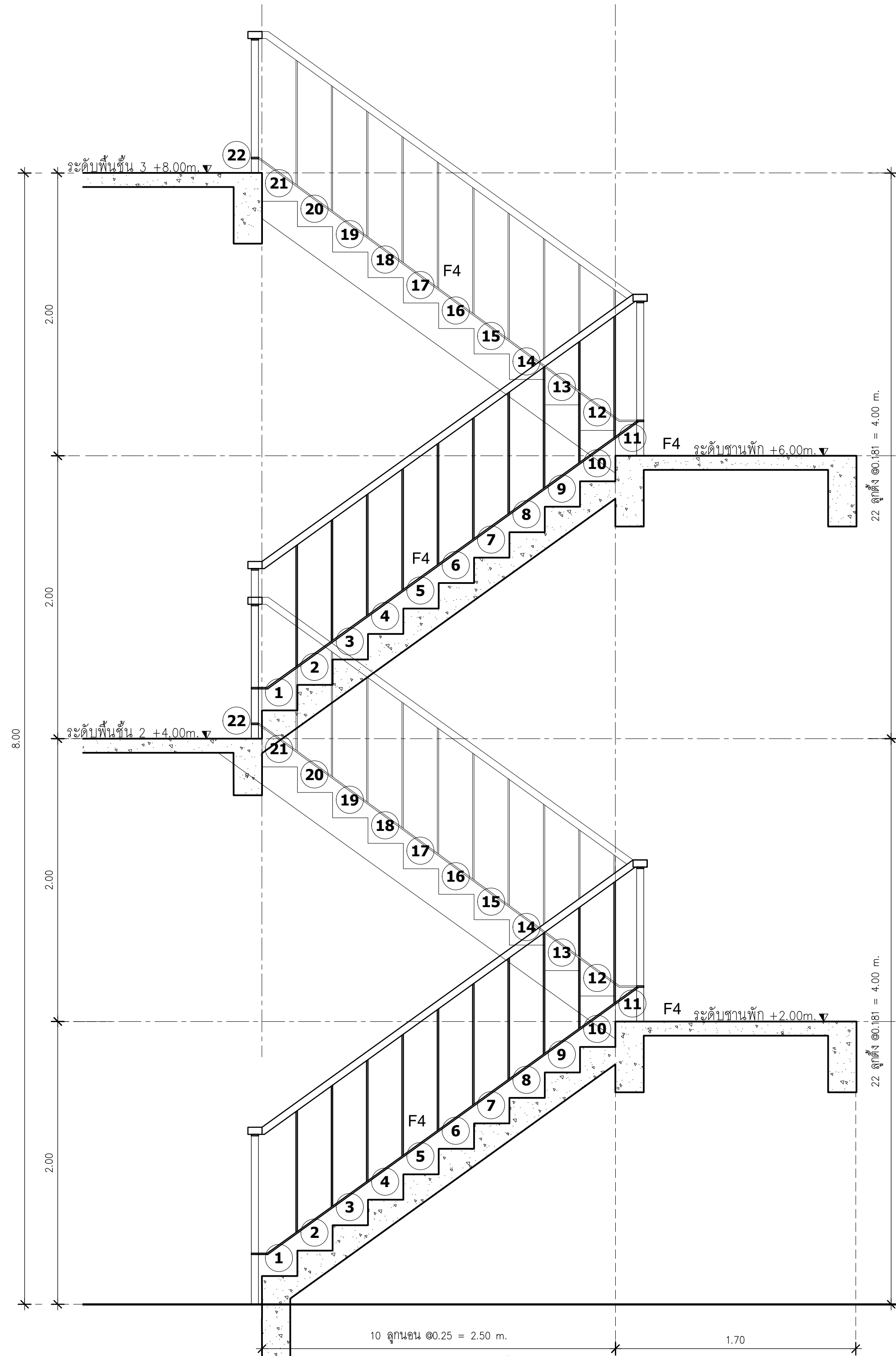
รูปตัดขยายบันได ST-8
