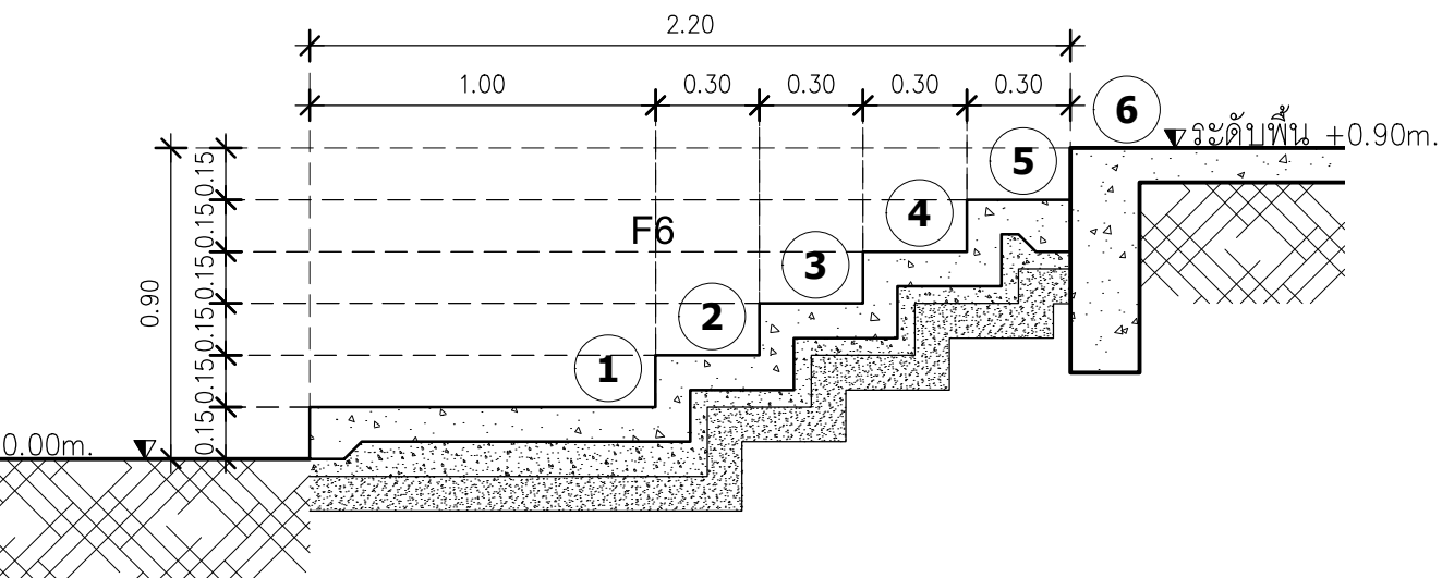
รูปตัดขยายบันได ST-9
