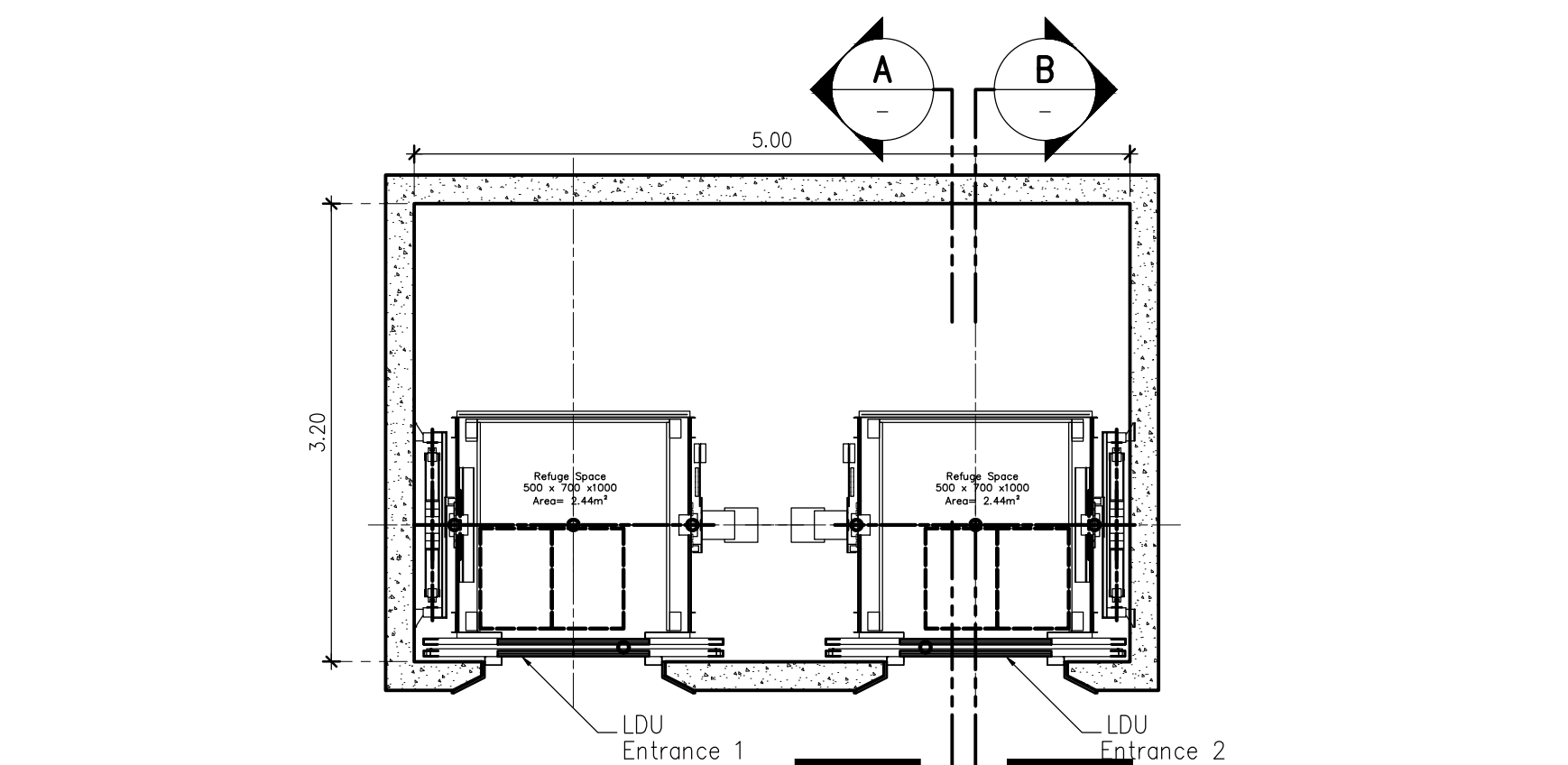
แปลนขยายลิฟท์
