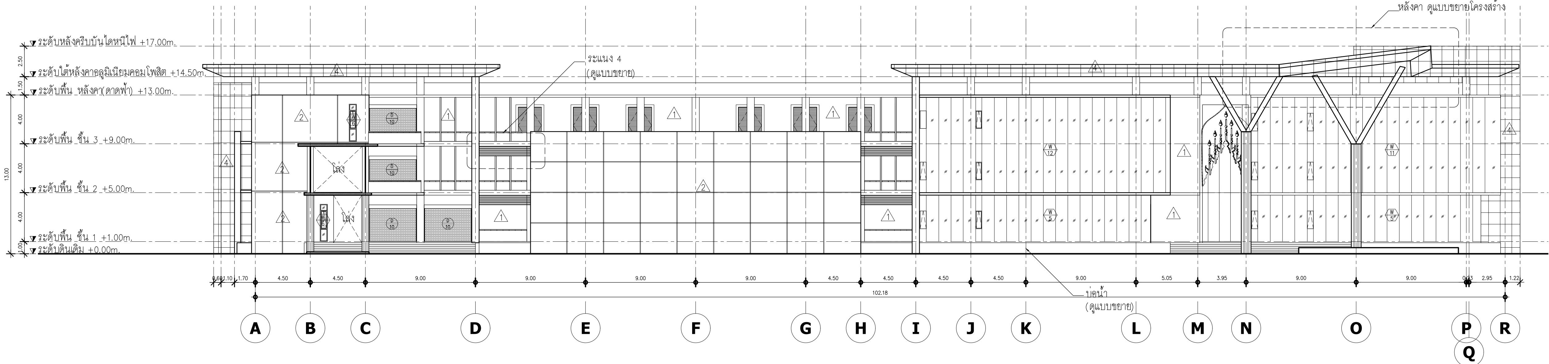
รูปด้าน 3 อาคาร A (บริหาร)
