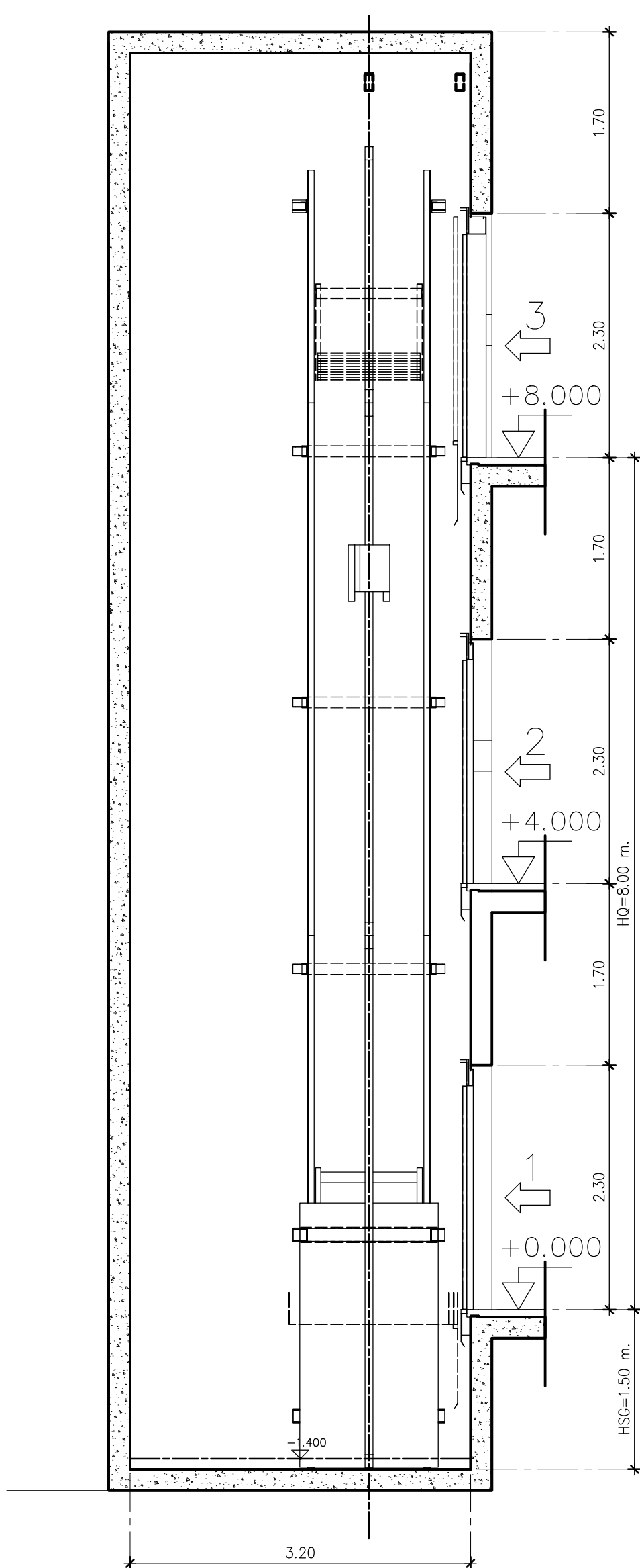
แปลนขยายลิฟท์ B
