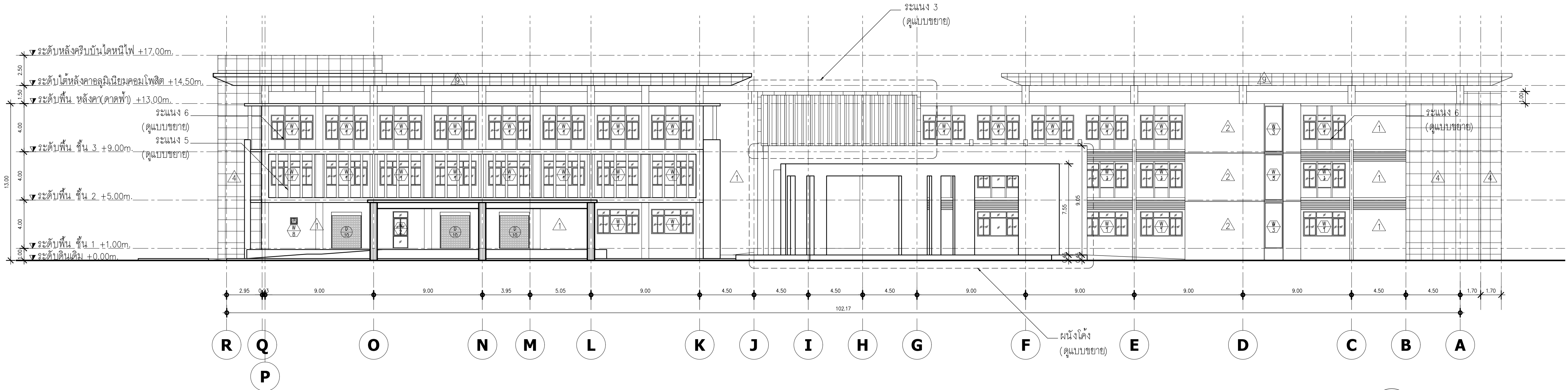
รูปด้าน 1 อาคาร A (บริหาร) SCALE 1:200
