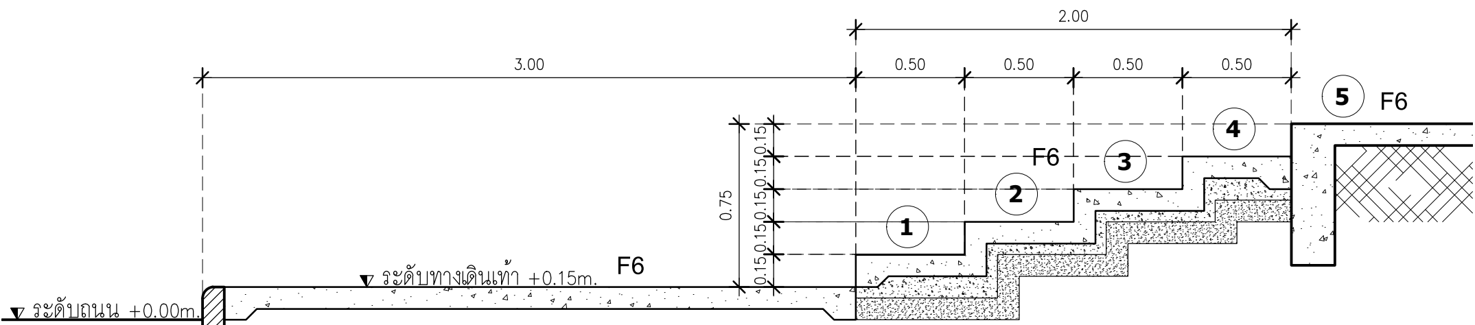
รูปตัดขยายบันได ST-11
