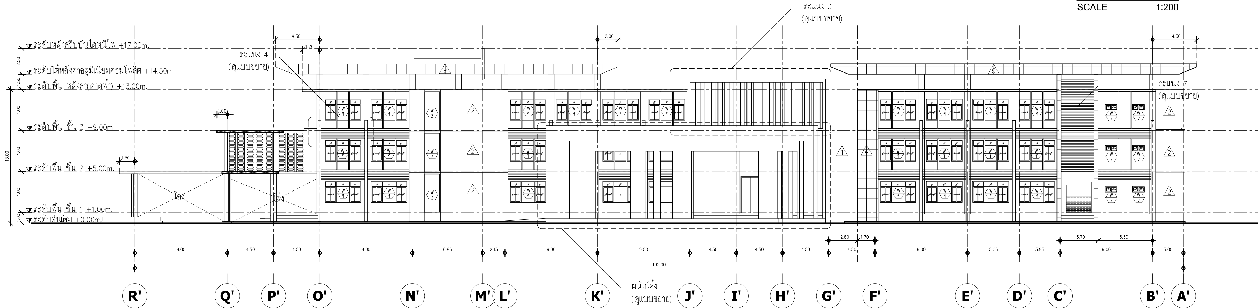
รูปด้าน 1 อาคาร B (บริการ)
