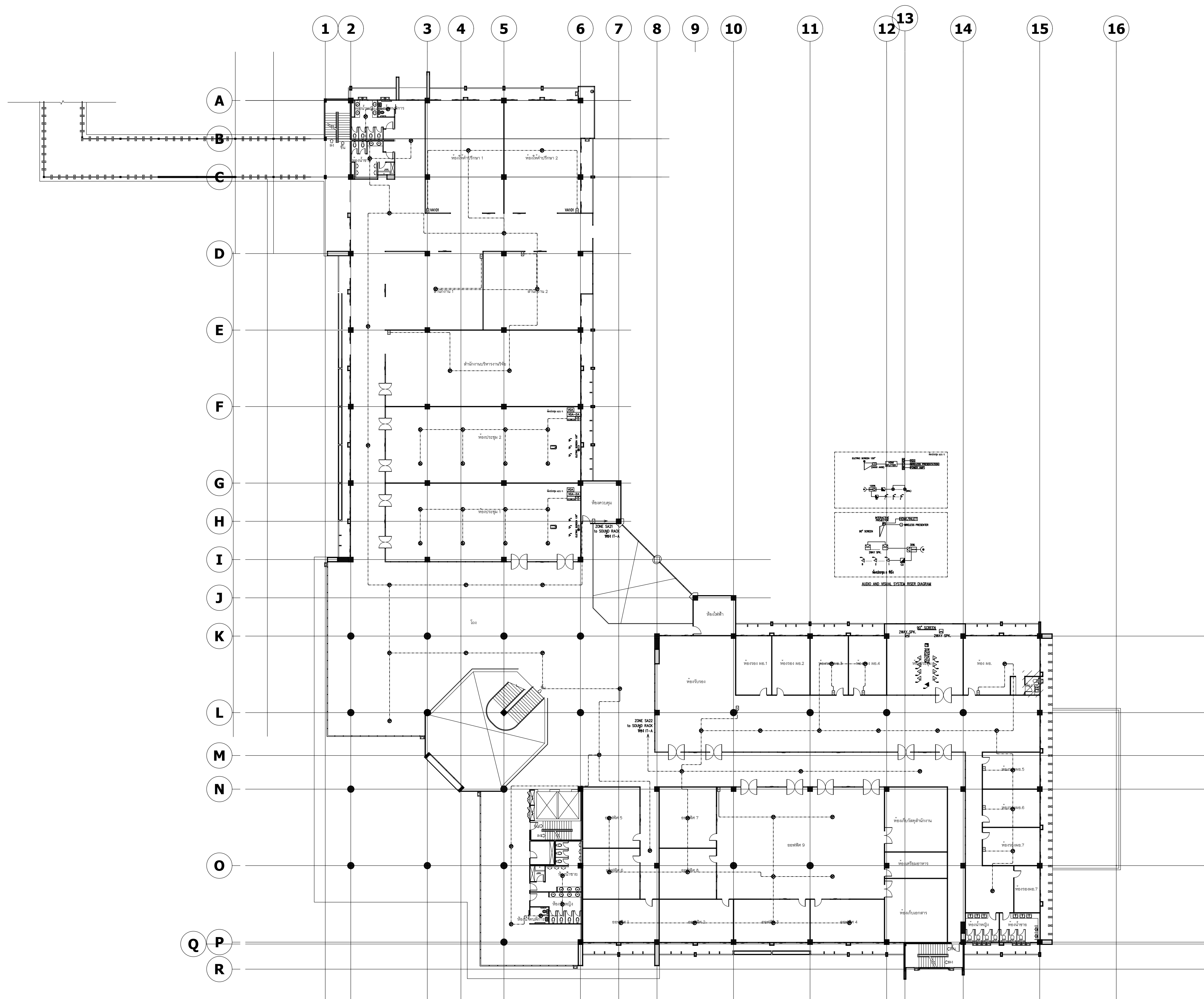
แปลนระบบเสียงประกาศ ชั้นที่ 2 อาคาร A (บริหาร)
