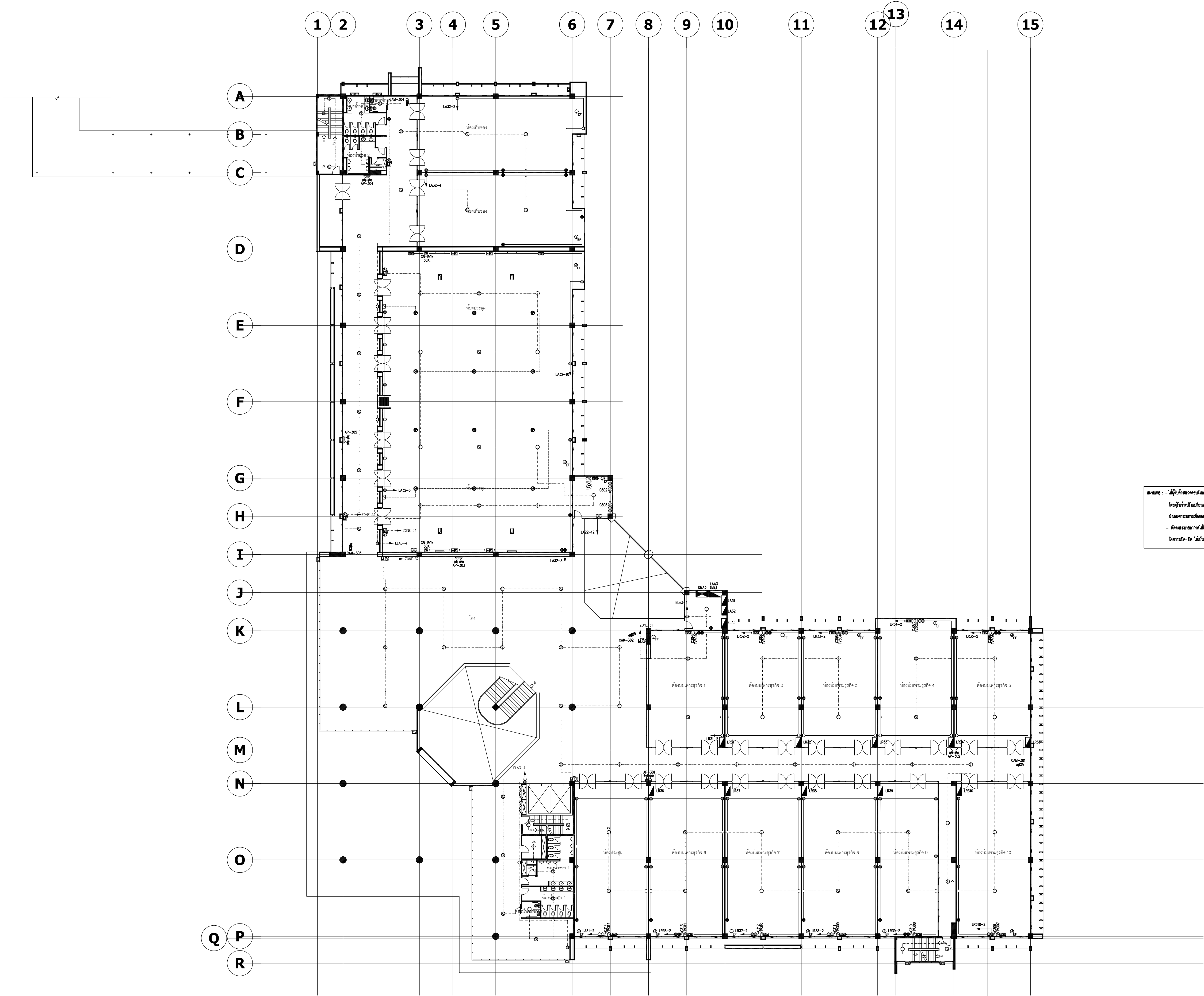
แปลนระบบไฟฟ้ากำลังและสื่อสาร ชั้นที่ 3 อาคาร A (บริหาร)
